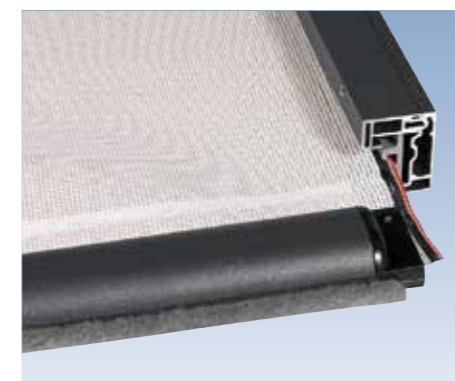
Seitensaumführung durch „Reißverschluss-Prinzip“
